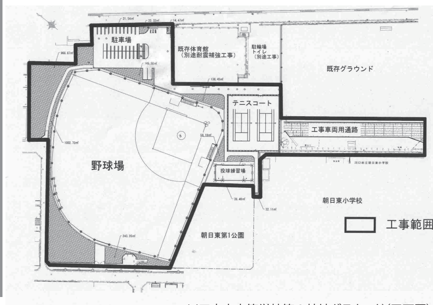
川口市立高等学校第2校地グラウンド（平面図）
